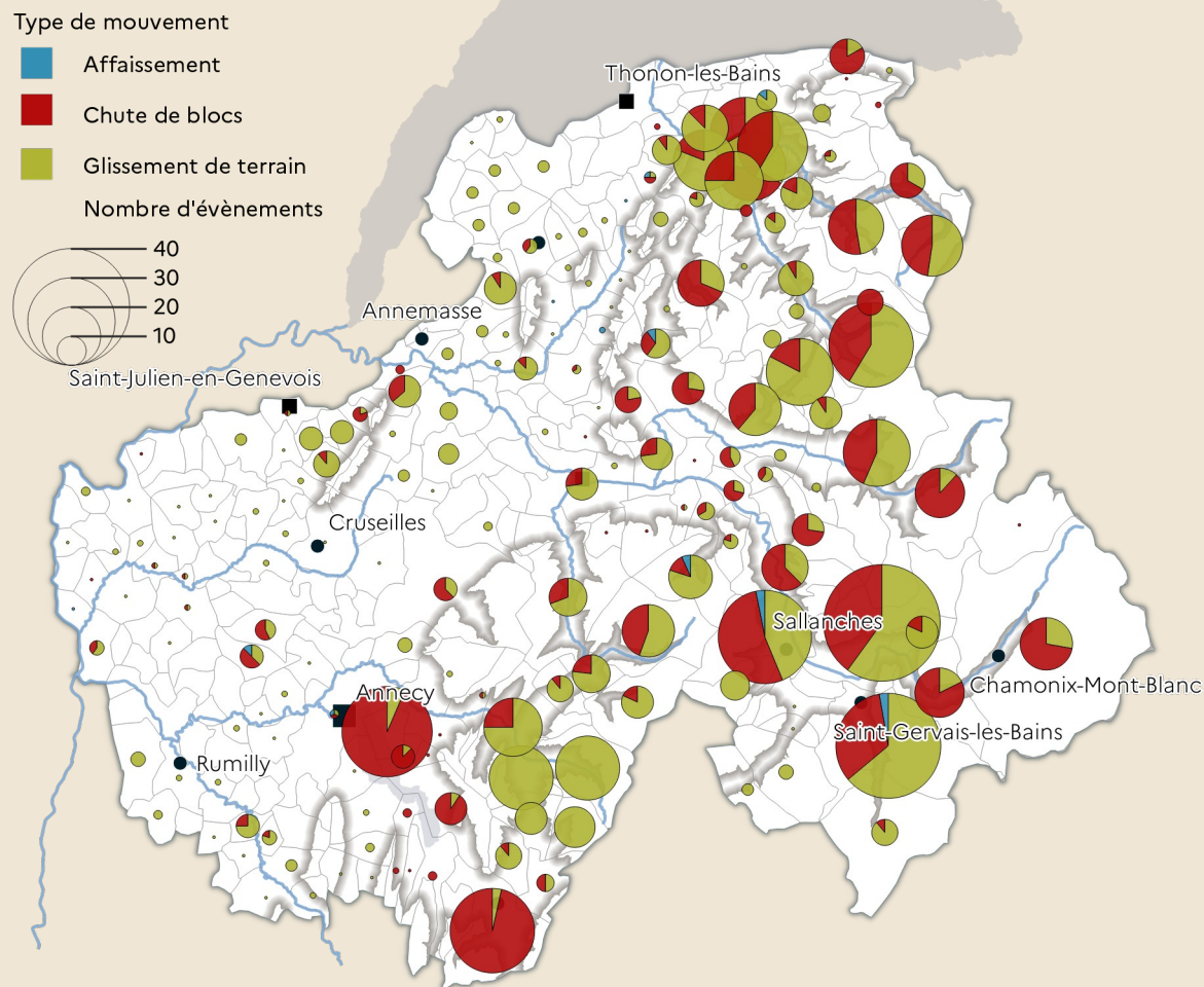
Carte départementale de l'histoire des mouvements de terrain source : ONF BD-RTM Événements de 1900 à 2019
