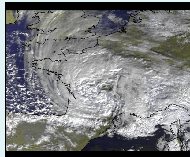
La tempête du 24 janvier (24/01/2009 à 09h45 UTC Satellite METOP2)
